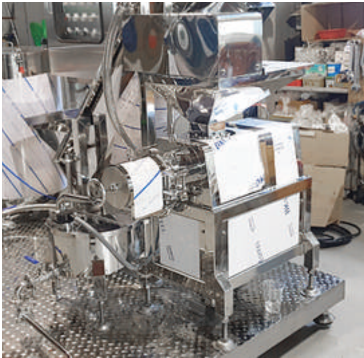
세척된 원물을 착즙하여 수위조절탱크로 이송하는 착즙기
